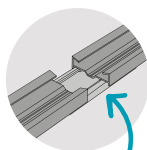
Jonctions Aluminium rail connection Schienenkonformes Aluminium Conexión ferroviaria de aluminio
