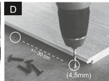
Foret de 4,5mm Boor een gat van 4,5mm
