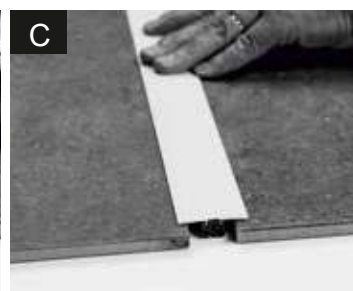
Maintenir pour la prise de la colle Druk het profiel goed aan zodat de kit zich kan verdelen
