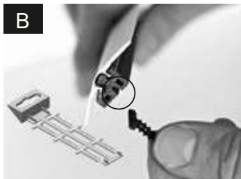
Insérer et glisser les vis Bevestig de schroeven
