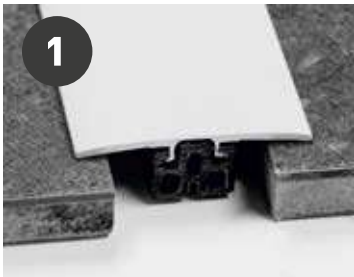
Profil de jonction Dilatatie profiel
