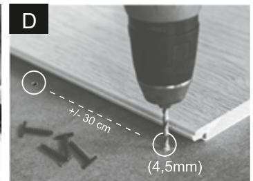
Foret de 4,5mm Boor een gat van 4,5mm
